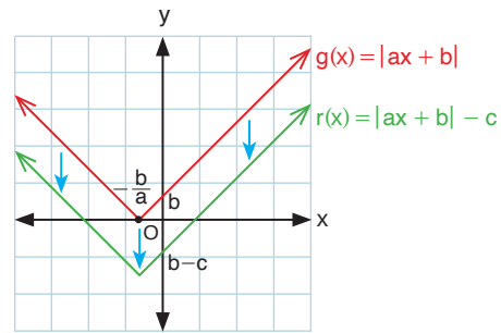
Grafik 2.9: r fonksiyonunun grafik temsili ( a, b, c \in \mathbb{R}^+ )
