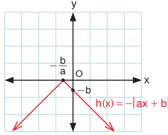
Grafik 2.7: h fonksiyonunun grafik temsili ( a, b \in \mathbb{R}^+ )
