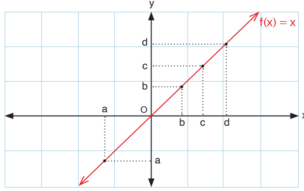
Grafik 2.2: f fonksiyonunun bire bir olduğunun gösterimi
