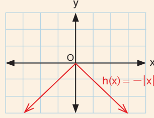
Grafik 2.4: h fonksiyonunun grafik temsili
