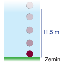
Görsel 1.3: Belirli bir yükseklikten bırakılan cisim
