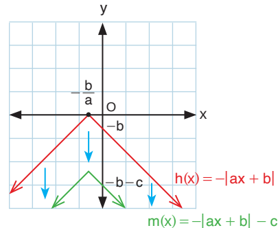
Grafik 2.11: m fonksiyonunun grafik temsili ( a, b, c \in \mathbb{R}^+ )
