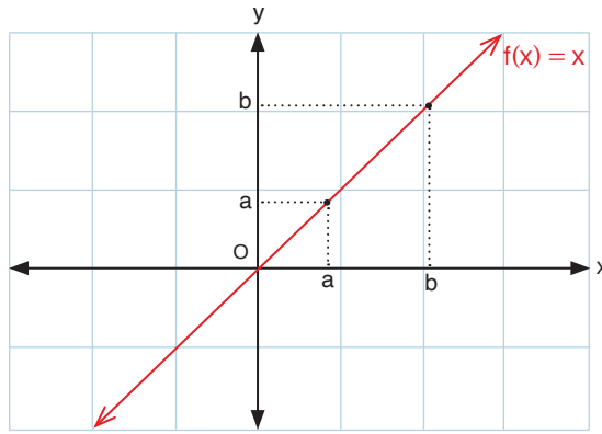
Grafik 2.1: f fonksiyonunun artanlığının gösterimi
