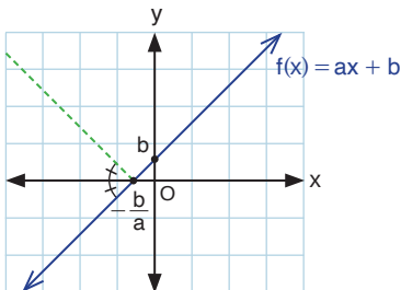
Grafik 2.5: f fonksiyonunun grafik temsili ( a, b \in \mathbb{R}^+ )
