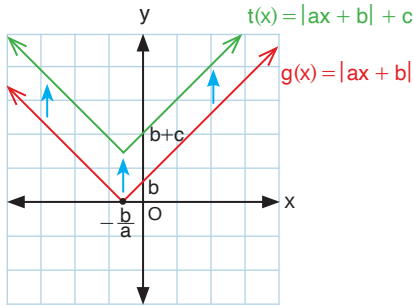
Grafik 2.8: t fonksiyonunun grafik temsili ( a, b, c \in \mathbb{R}^+ )
