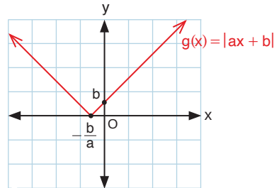
Grafik 2.6: g fonksiyonunun grafik temsili ( a, b \in \mathbb{R}^+ )
