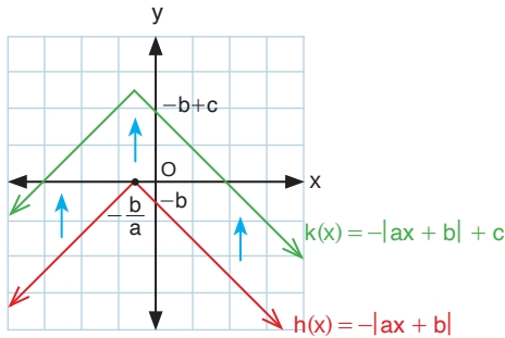
Grafik 2.10: k fonksiyonunun grafik temsili ( a, b, c \in \mathbb{R}^+ )
