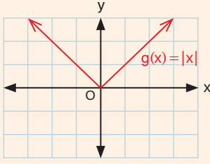
Grafik 2.3: g fonksiyonunun grafik temsili
